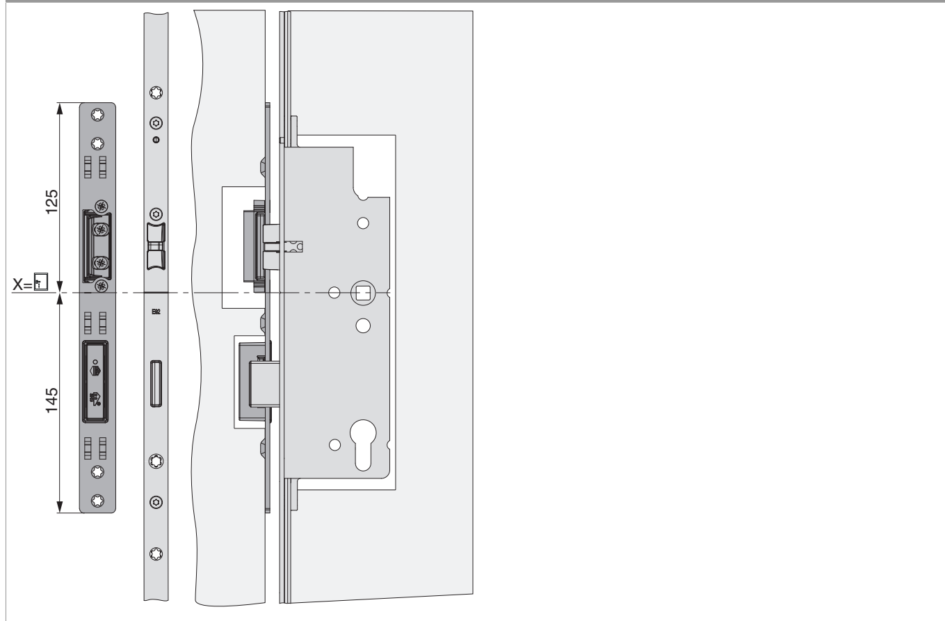
Fallen- und Riegelschließteile
