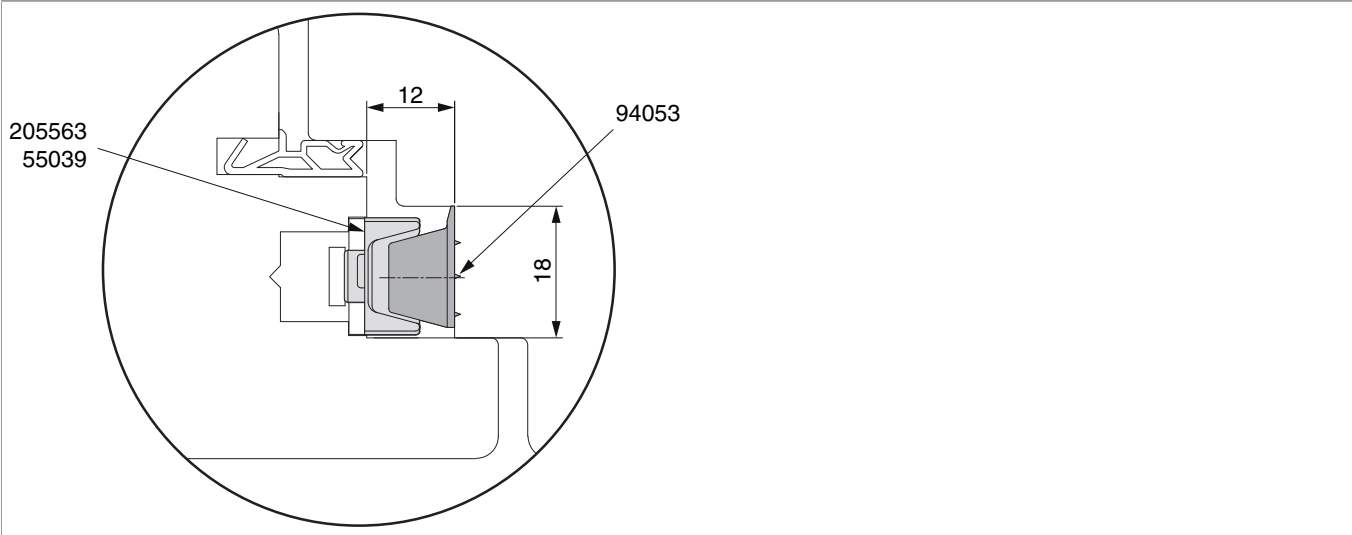
Detailansicht mit Schließzapfen Eurofalz
