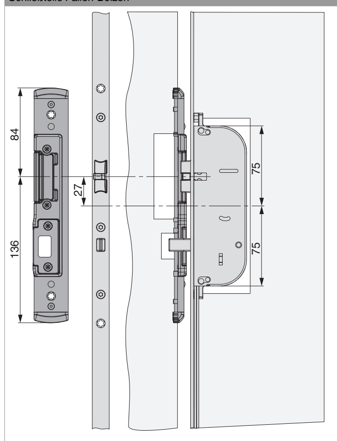
Schließteile Fallen-Bolzen
