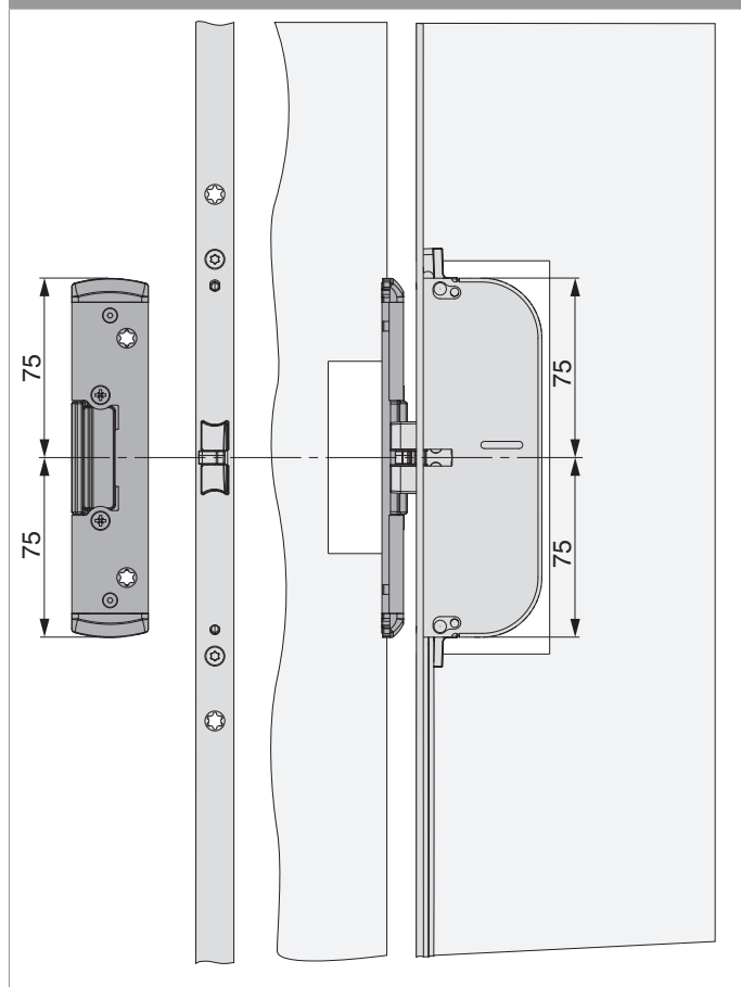
Schließteile Fallen-Bolzen
