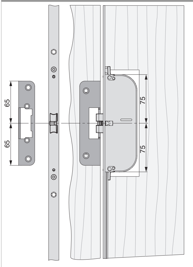
Winkelschließblech Falle
