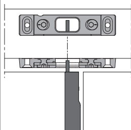
2-Flg. Tür mit 1 Riegel
