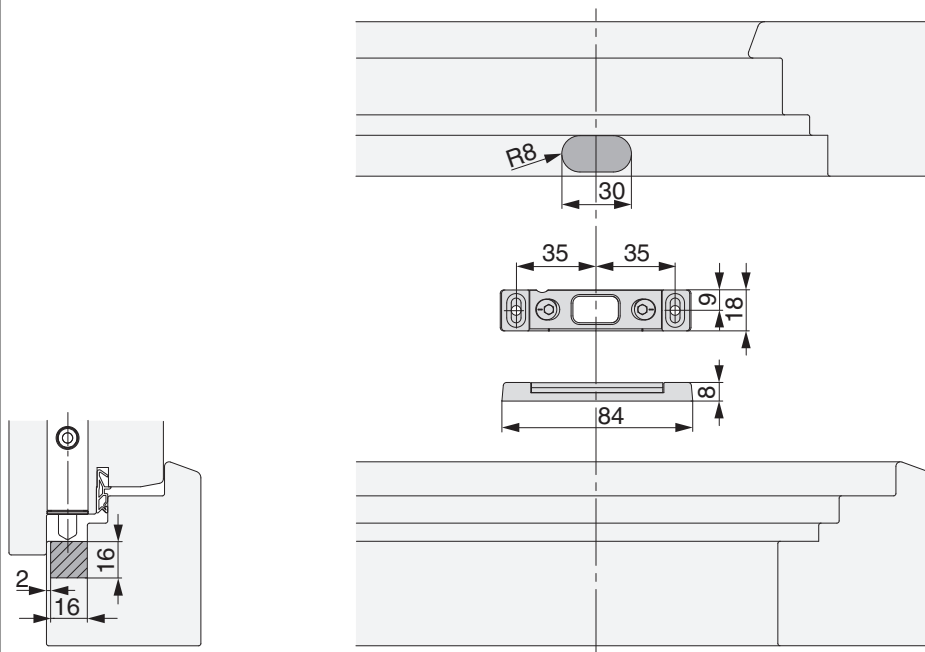
Riegelschließteile
