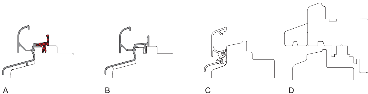
A = Thermisch getrennt, klemmbar. B = keine thermische Trennung, klemmbar. C = Regenschutzschiene, vorgesetzt/geklippt. D = Wetterschenkel
