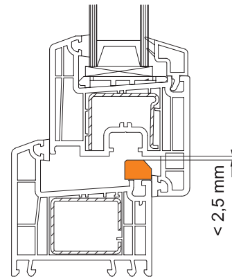
Bild 1: Position des Auflaufes, Luft zwischen Auflauf und Flügelfalzante
