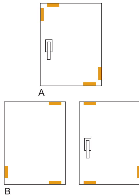
Bild 2: A = Position der Aufläufe bei einflügeligen Fenstern. B = Position der Aufläufe bei zweiflügeligen Fenstern.
