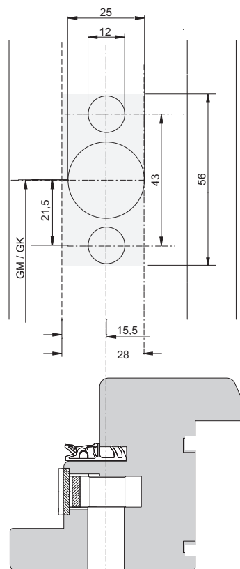
Bild 3: Ermittlung des Dornmaßes
