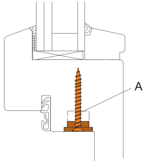
Bild 1: A = Beschlagschraube 4x35 mm, 2 mm vorgebohrt
