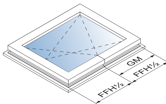
Bild 1 : Flügelalzhöhe FFH mit mittigem Griffsitz
