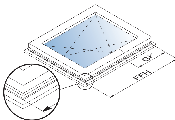
Bild 2 : Flügelalzhöhe FFH mit konstantem Griffsitz
