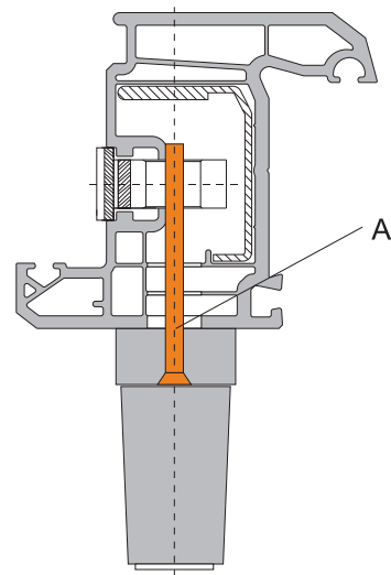
Befestigung der Sicherheits-Griffolive A = Schrauben M5, Länge abstimmen und Profilsituation
