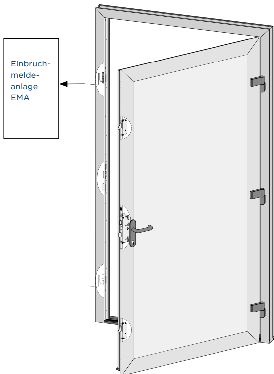
Abbildung 3-1: Haustür mit Verriegelung autoLock AV3 und Riegel-Schalt-Kontakt RSK MV/UMV an Schwenkriegel-Tasche (Empfohlene Einbau-Position: Oberes Nebenverriegelungselement)
