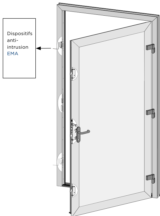
Figure 3-1: Porte avant à verrouillage autoLock AV3 et contact de commutation à pêne RSK MV/UMV sur pochette à verrou crochet (Position d'installation recommandée: Élément de verrouillage du côté supérieur)
