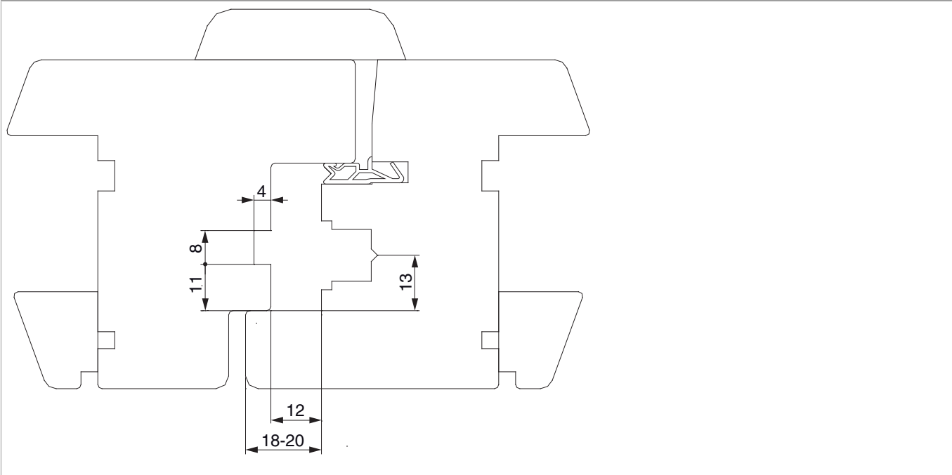
alternative Fensterkonstruktion 2flg.
