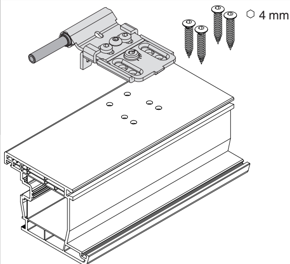
Verschraubung Türband an der Tür
