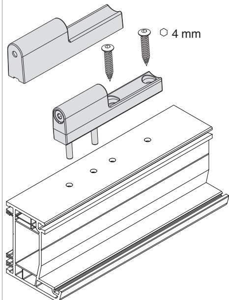
Einführung des Stiftes ins Türband
