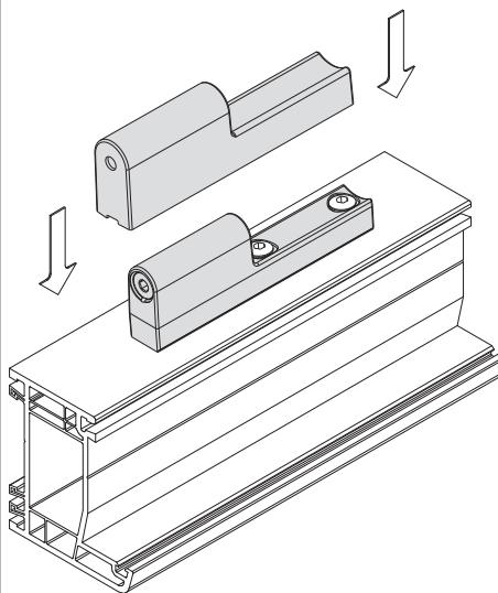
Befestigung der Türbandabdeckung
