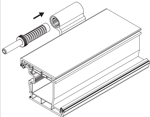
Montage Achsstift
