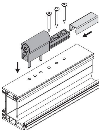
Montage Rahmenteil
