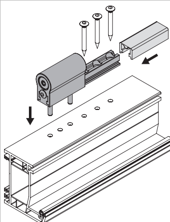
Montage Rahmenteil
