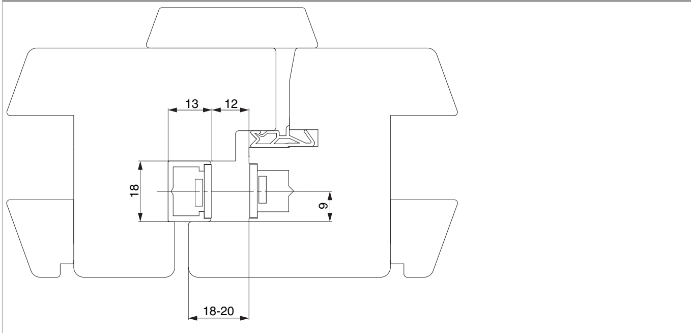
Gegenüberliegende Beschlagsnut mit Alukanal
