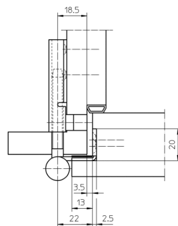
Querschnitt
