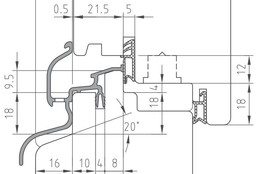
Einbaubeispiel RDN 22.45 K Installation example
