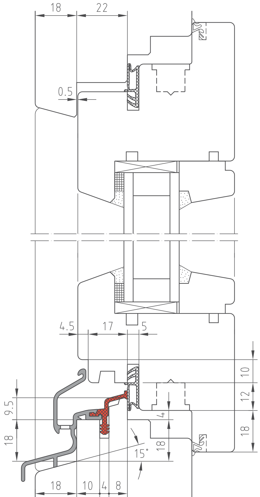
Einbaubeispiel TRD 22.46 K Installation example
