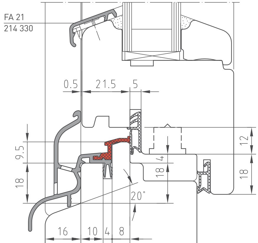
Einbaubeispiel TBSDN 22 K Installation example
