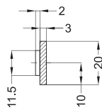
D - D
