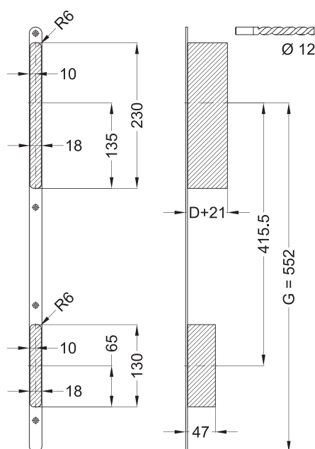
Fräsmaße
