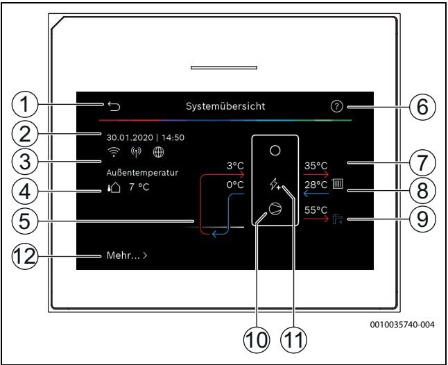
Bild 7 Anlagenübersicht
