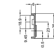
Allgemeine Vermaßung
