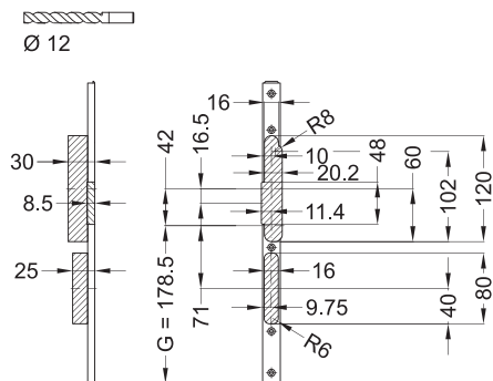
Fräsmaße
