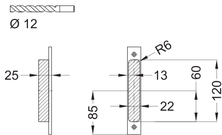
Fräsmaße
