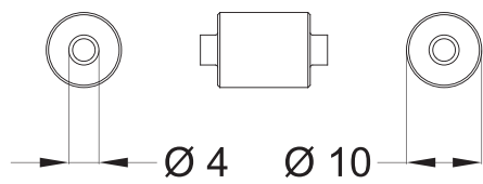
Ansichten
