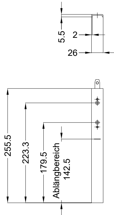
T-ASS-A U26 BN13-5,5-256 NL
