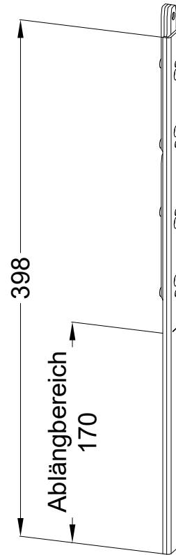
T-ASS-A U26 BN13-5,5-399-1 NL
