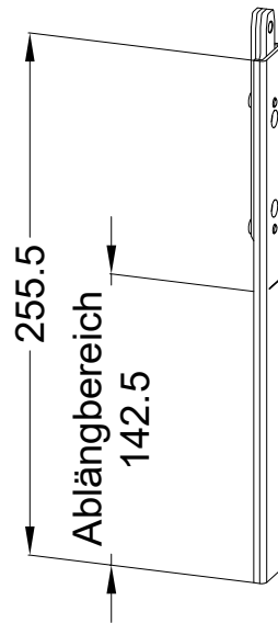
T-ASS-A U26 BN13-5,5-256 NL
