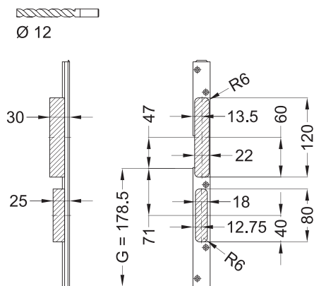
Fräsmäße
