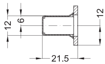
C - C
